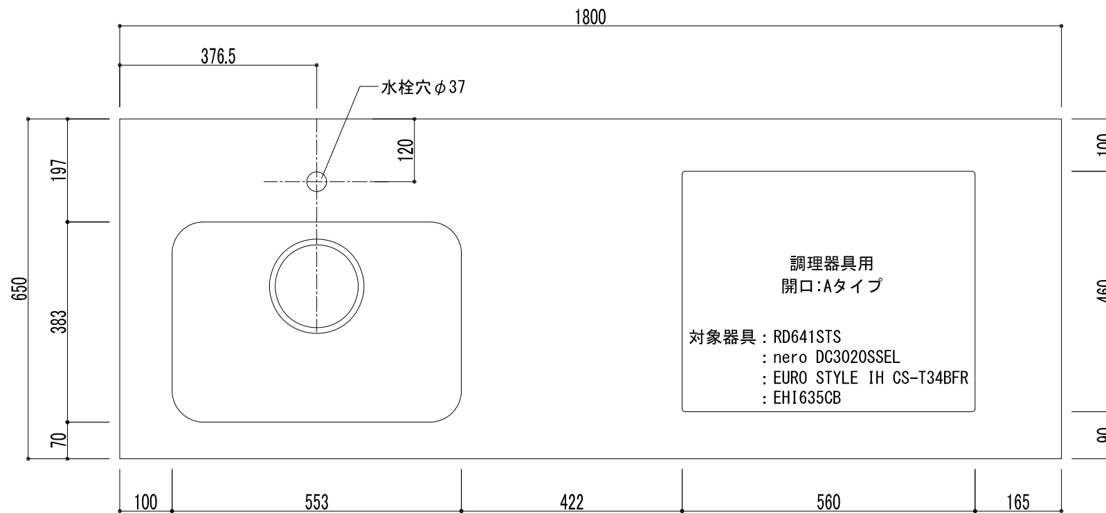
平面図
