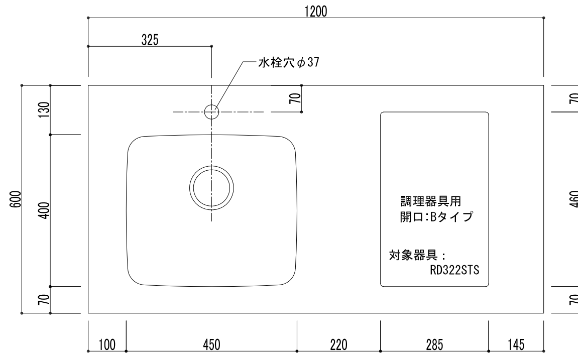
平面図
