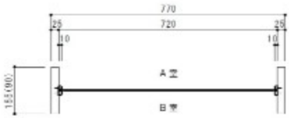
下段 ヨコ断面図
