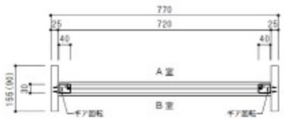
上段 ヨコ断面図
