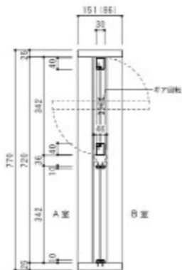
タテ断面図
