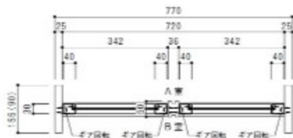
上段 ヨコ断面図
