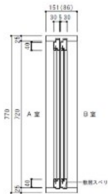
タテ断面図
