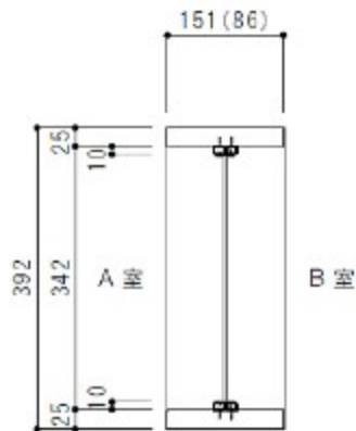
タテ断面図 FIX窓
