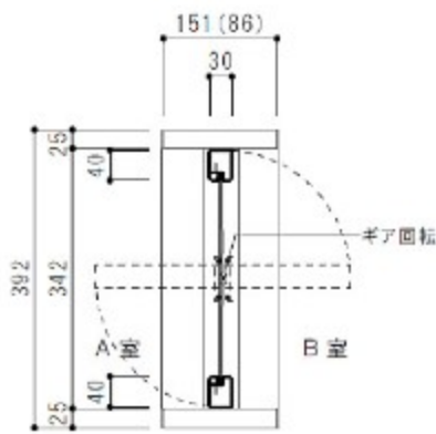
タテ断面図 横軸回転窓
