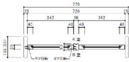
ヨコ断面図
