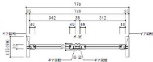
ヨコ断面図
