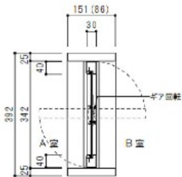
タテ断面図
