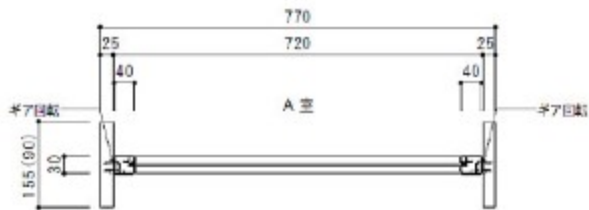
ヨコ断面図
