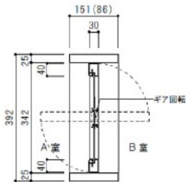
タテ断面図
