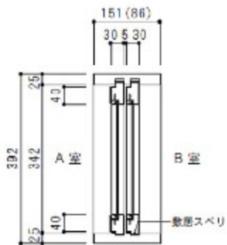
タテ断面図
