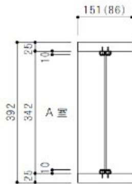
タテ断面図
