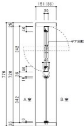
タテ断面図
