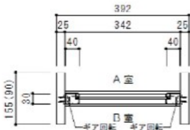
ヨコ断面図
