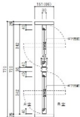
タテ断面図
