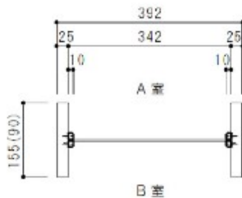
ヨコ断面図
