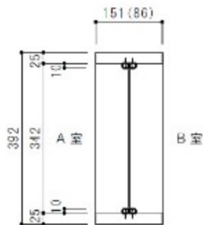
夕テ断面図
